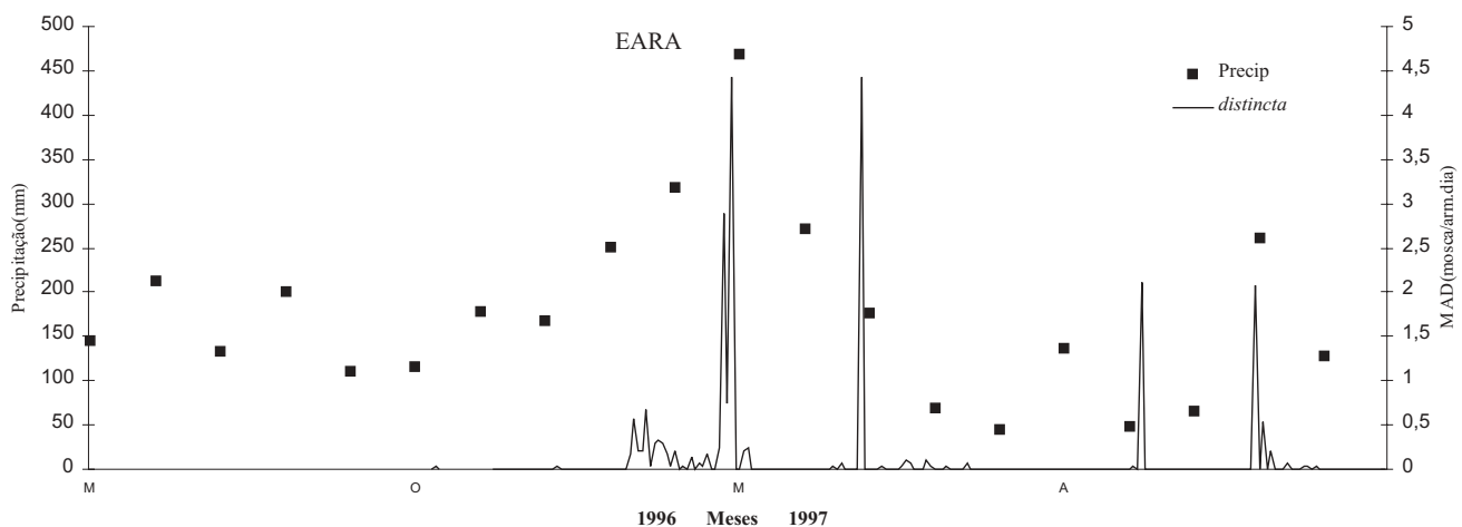
Fig. 4. Flutuação populacional de A. distincta capturadas em armadilhas McPhail e a precipitação pluviométrica na EARA, BR 174 km 23, Manaus, AM, de maio de 1996 a dezembro de 1997.
