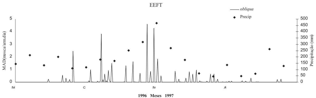
Fig. 8. Flutuação populacional de A. obliqua capturada em armadilhas McPhail e a precipitação pluviométrica na EEFT, INPA, BR 174, km 40, Manaus, AM, de maio de 1996 a dezembro de 1997.
