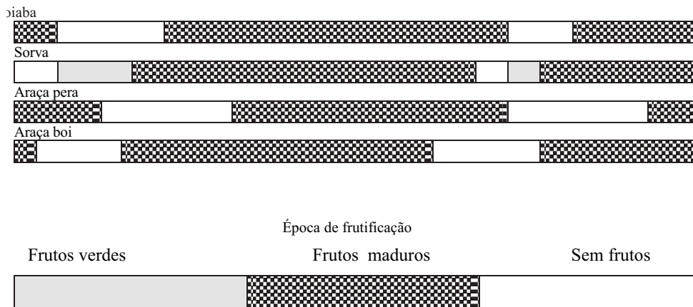
Fig. 7. Flutuação populacional de Anastrepha spp. na EEFT, INPA, BR 174, km 23, Manaus, Am, no período de maio de 1996 a dezembro de 1997.
