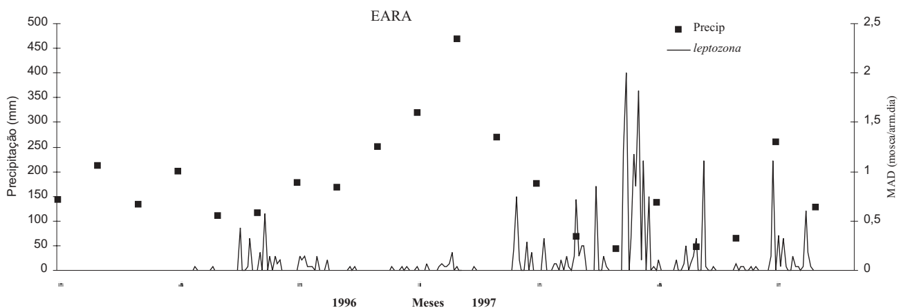
Fig. 5. Flutuação populacional de A. leptozona capturadas em armadilhas McPhail e a precipitação pluviométrica na EARA, BR 174, km 23, Manaus, AM, de maio de 1996 a dezembro de 1997.
