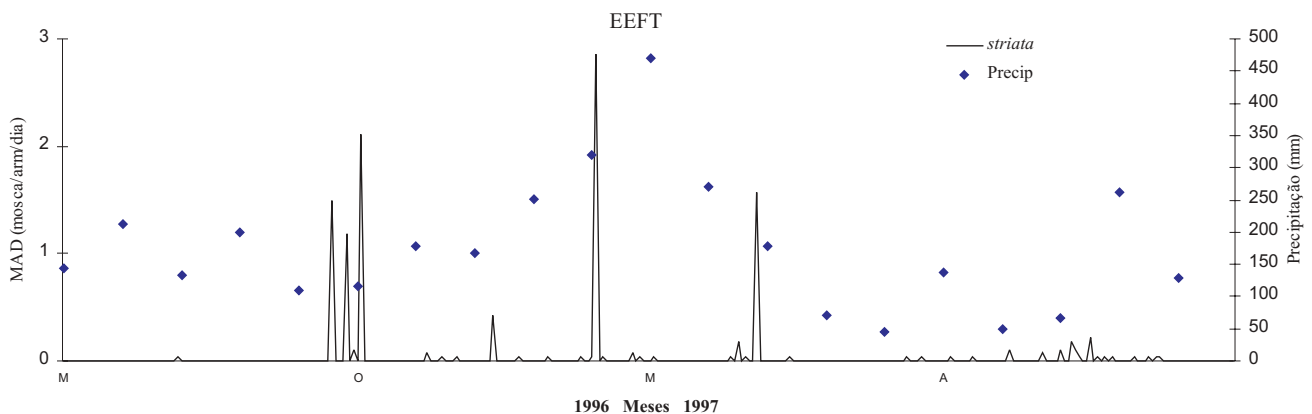
Fig. 9. Flutuação populacional de A. striata capturadas em armadilhas McPhail e a precipitação pluviométrica na EEFT, INPA, BR 174, km 40, Manaus, Am, de maio de 1996 a dezembro de 1997.
